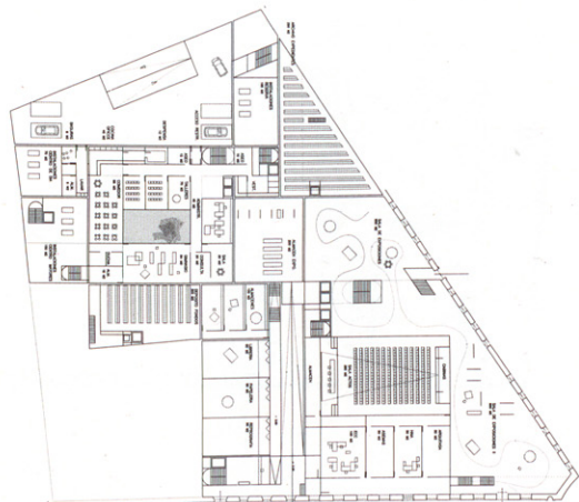
PLANTA SEMISÓTANO
